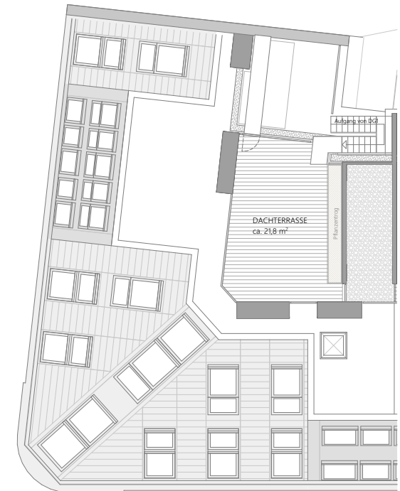
Dachdraufsicht
