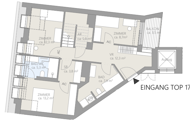
1. Dachgeschoss
